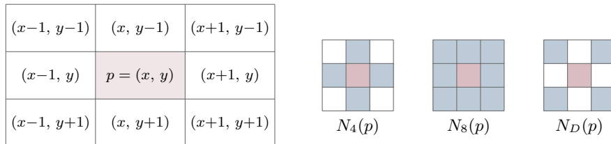
Figura 2.7. I 4-vicini, gli 8-vicini e i vicini diagonali del pixel p .
