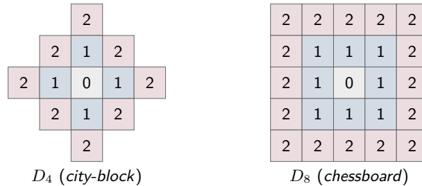
Figura 2.9. Distanze D_4 e D_8 dal pixel centrale, fino a 2.
