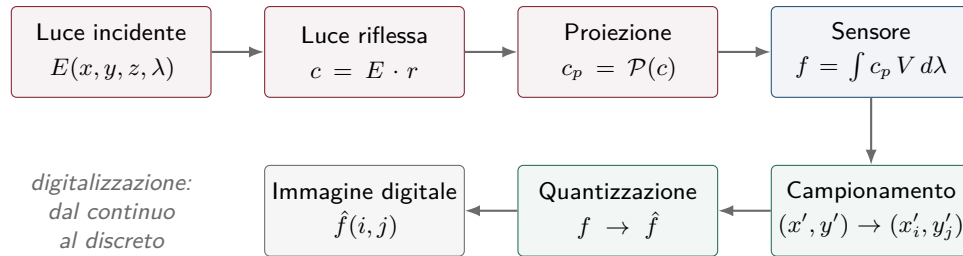
Figura 2.3. La catena che porta dalla luce incidente all'immagine digitale. Nella prima riga la formazione dell'immagine, ancora continua; nella seconda la digitalizzazione.
