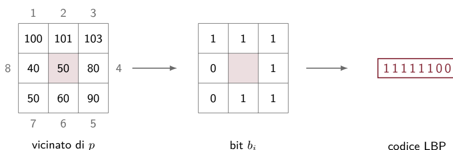
Figura 3.8. Calcolo del codice LBP del pixel centrale. I numeri in grigio indicano l'ordine dei vicini.
