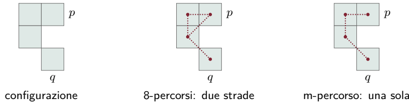
Figura 2.8. Percorsi da p a q . Con l'8-adiacenza il primo passo può tagliare in diagonale oppure passare per il pixel a sinistra di p . Con l'm-adiacenza quel taglio non è ammesso, perché il pixel a sinistra di p è un 4-vicino comune della stessa classe, e il percorso è unico.
