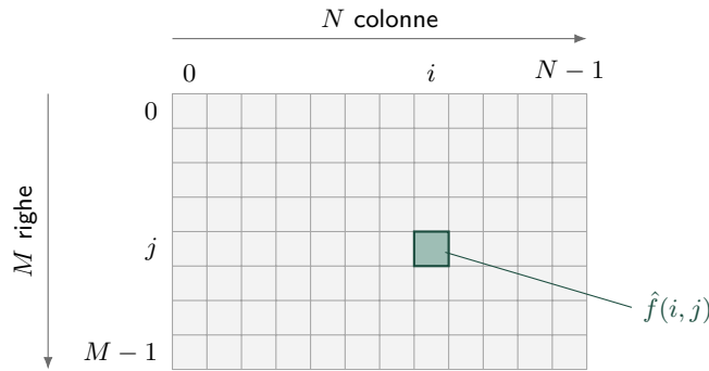
Figura 2.6. Un'immagine come array di M righe e N colonne.
