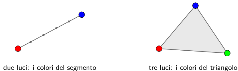
Figura 3.4. In uno spazio colore lineare le miscele di due luci stanno sul segmento che le unisce, quelle di tre luci nel triangolo che definiscono.
