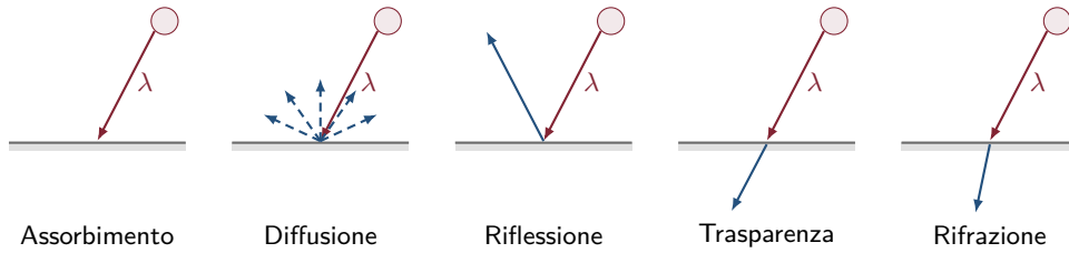
Figura 2.1. Che cosa può succedere alla luce di lunghezza d'onda \lambda quando incontra una superficie.
