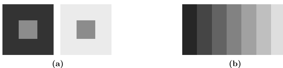
Figura 3.7. (a) Contrasto simultaneo: i due quadrati centrali hanno lo stesso grigio, ma su sfondo scuro sembra più chiaro. (b) Bande di Mach: ogni fascia è uniforme, ma vicino a ogni bordo sembra più chiara dal lato chiaro e più scura dal lato scuro.
