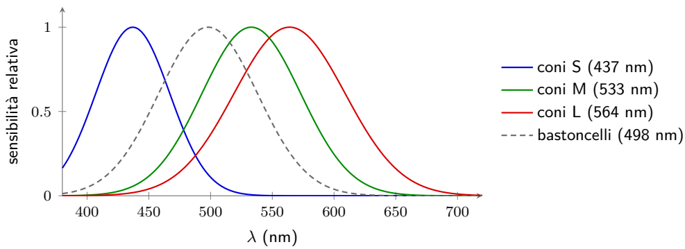
Figura 3.3. Sensibilità relative dei tre tipi di coni e dei bastoncelli (curve indicative).
