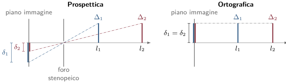
Figura 2.2. Due oggetti uguali a distanze diverse. Con la proiezione prospettica il più lontano ha un'immagine più piccola ( \delta_2 < \delta_1 ), con quella ortografica le immagini sono uguali.
