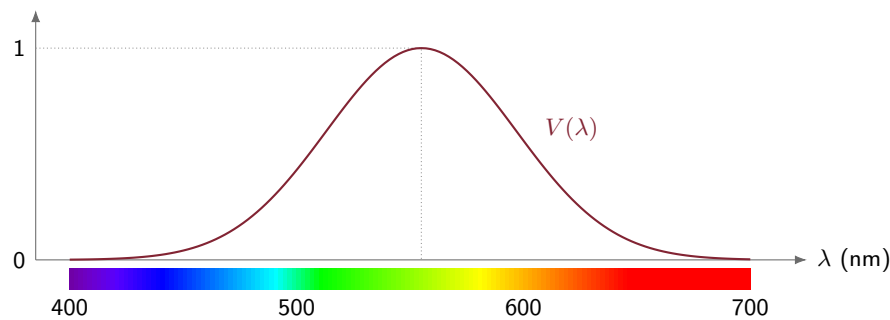
Figura 3.1. Lo spettro visibile e la sensibilità dell'occhio alla luminanza V(\lambda) (curva indicativa).
