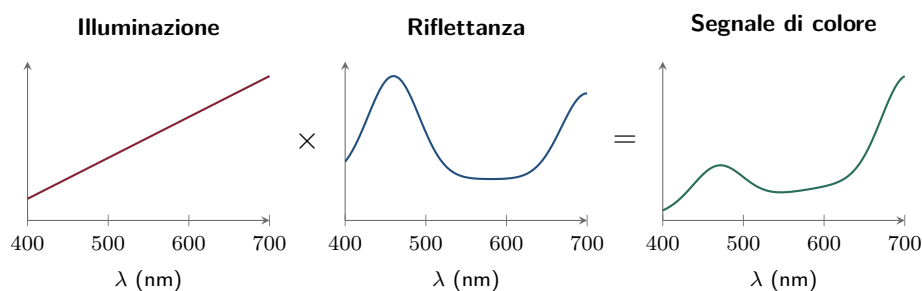
Figura 3.2. Il segnale di colore è il prodotto, lunghezza d'onda per lunghezza d'onda, dello spettro dell'illuminazione e della riflettanza della superficie (curve indicative).
